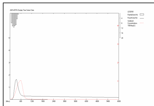
Gambar 9 Grafik hidrograf dan konsentrasi sedimen akibat hujan.
