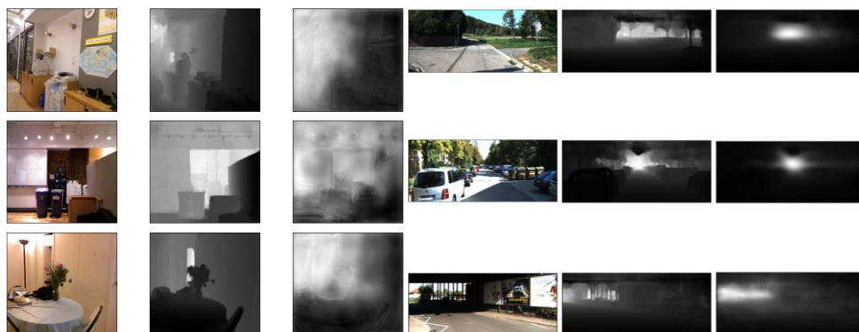
Gambar 4. (kiri) Keluaran dengan NYU Depth Dataset, (kanan) Keluaran dengan Kitti Dataset
