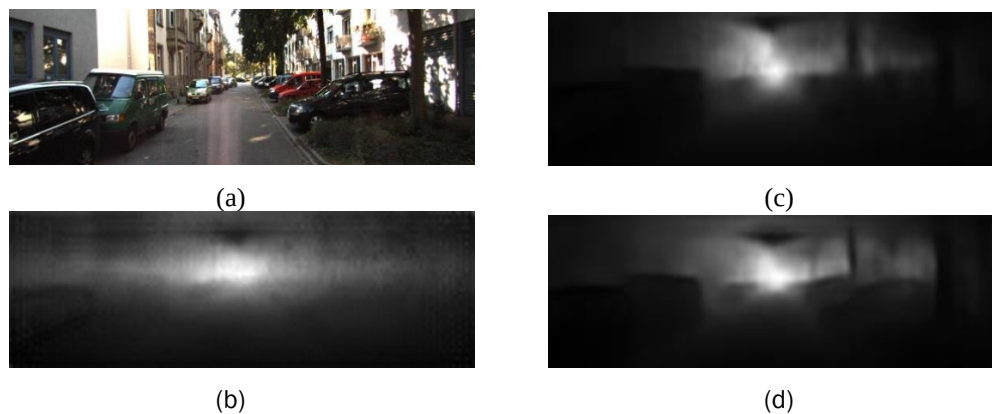
Gambar 7. Hasil pengujian penerimaan citra RGB tunggal (luar ruang) (a) citra masukan, (b) arsitektur 1., (c) arsitektur 2., (d) arsitektur 3.
