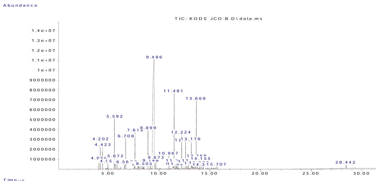
Gambar 1. Hasil kromatogram bahan baku
