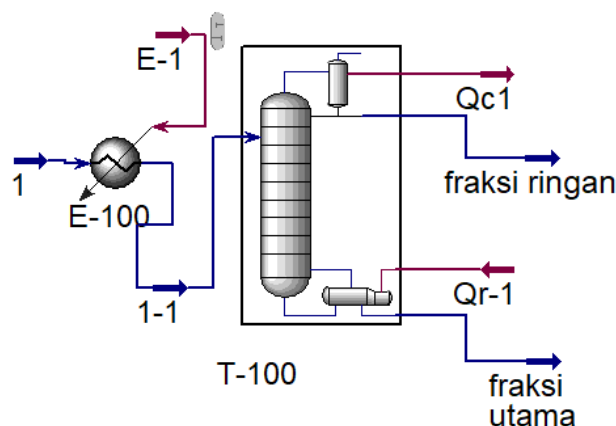
Gambar 2. Konfigurasi model proses.
