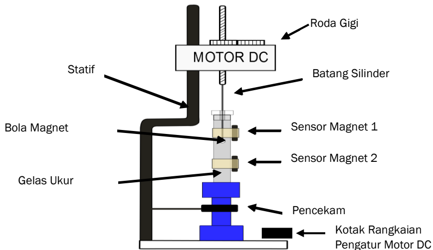
Gambar 4 Rancangan prototipe
