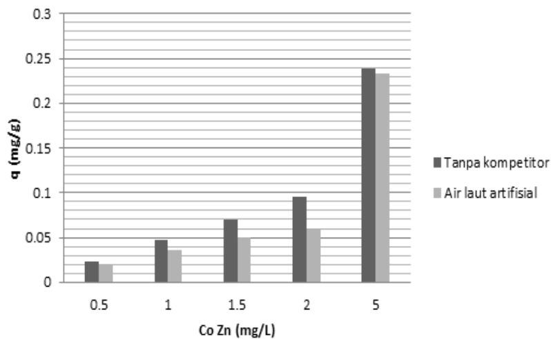
Gambar 6. Kapasitas adsorpsi Zn pada air laut artifisial dengan beberapa konsentrasi awal Zn pada waktu ekuilibrium
