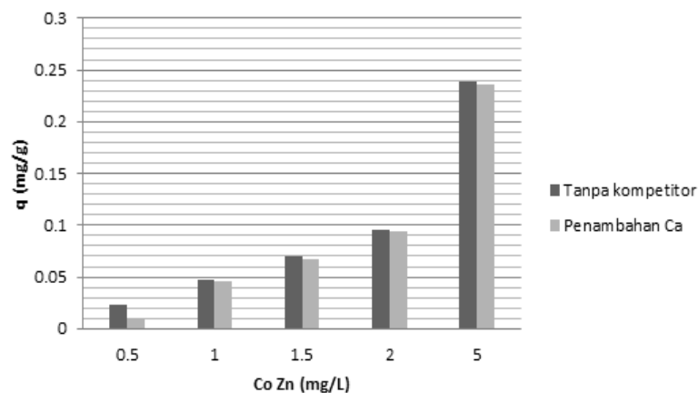
Gambar 4. Pengaruh penambahan Ca terhadap kapasitas adsorpsi Zn pada beberapa konsentrasi awal Zn pada waktu ekuilibrium
