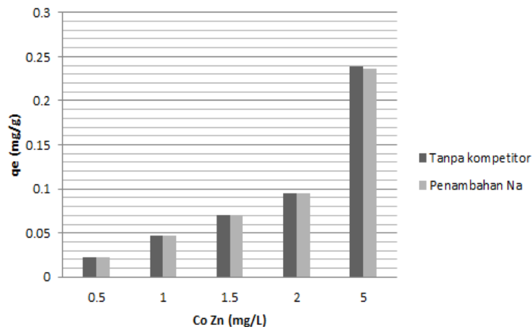
Gambar 3. Pengaruh penambahan Na terhadap kapasitas adsorpsi Zn pada beberapa konsentrasi awal Zn pada waktu ekuilibrium
