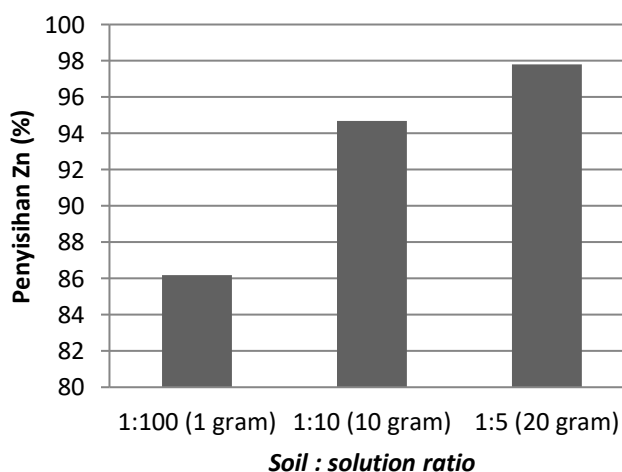
Gambar 2. Persentase penyisihan seng pada tiap dosis sorben
