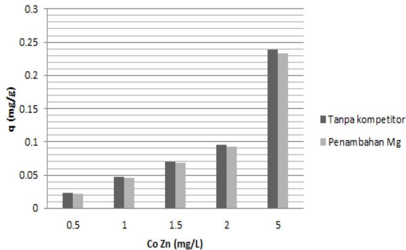
Gambar 5. Pengaruh penambahan Mg terhadap kapasitas adsorpsi Zn pada beberapa konsentrasi awal Zn pada waktu ekuilibrium
