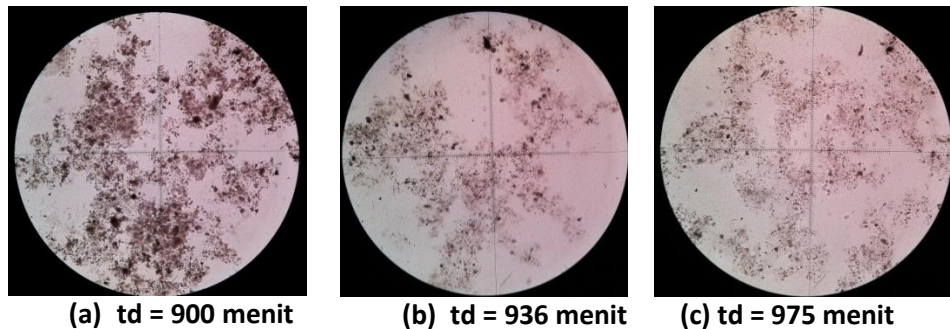
Gambar 8. Bentuk dan ukuran flok pada kerapatan arus 104 A/m 2 .
