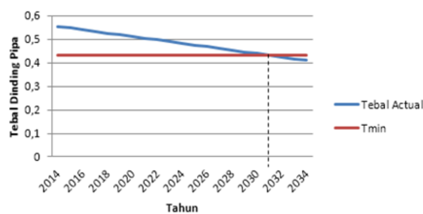
Gambar 7 Grafik Remaining Life Time pada Pipa Gas Lurus ( Outlet Automatic Shutdown Valve ) KP-20 Ø 20”.
