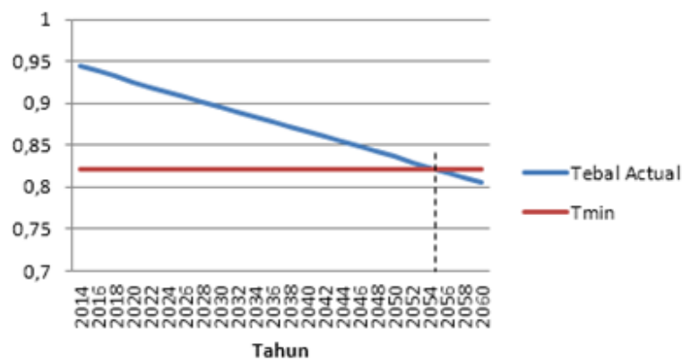
Gambar 6 Grafik Remaining Life Time pada Sambungan Tee (KP-20 Ø 20").
