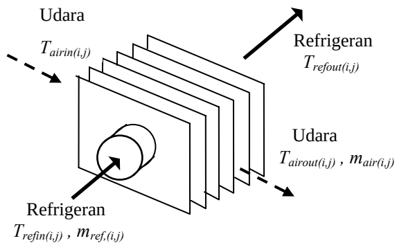
Gambar 2 Aliran fluida melalui sebuah elemen volume
