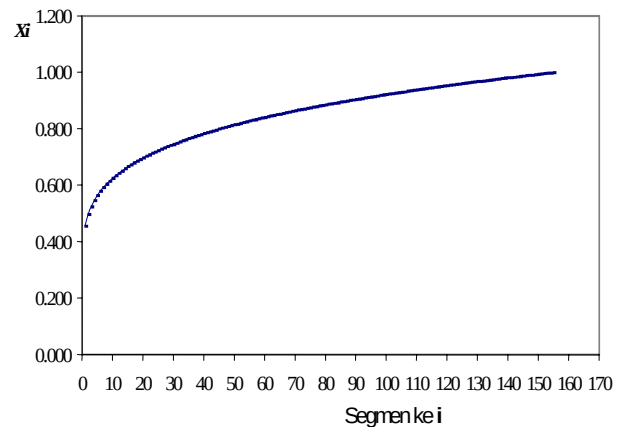
Gambar 8 Perubahan kualitas uap refrigeran sepanjang pipa.
