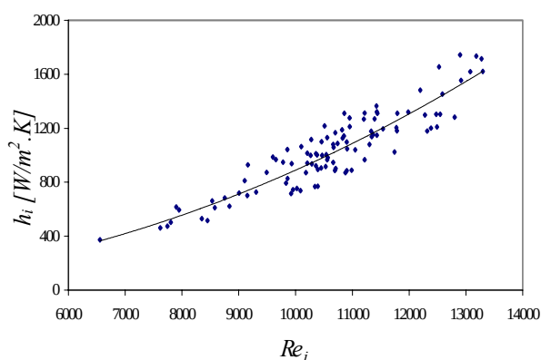
Gambar 6 Koefisien perpindahan panas di sisi refrigeran pada evaporator uji.
