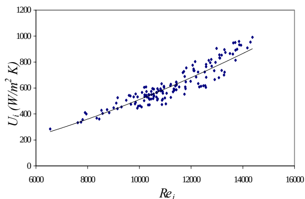
Gambar 5 Koefisien perpindahan panas keseluruhan (global) pada evaporator uji.
