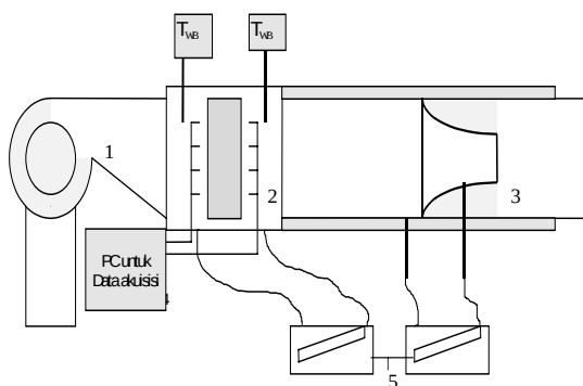
1. Blower, 2. Evaporator Uji, 3. Flow nozzle, 4. PC untuk akuisisi data, 5. Manometer
