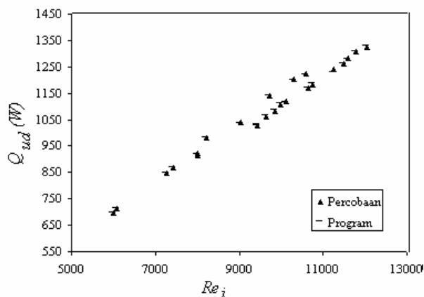
Gambar 7 Perbandingan antara hasil kaji numerik dan eksperimental evaporator uji.
