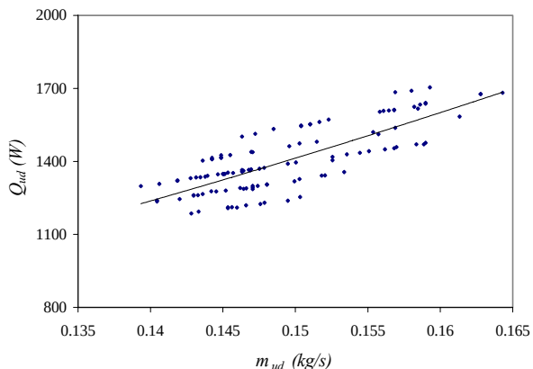
Gambar 4 Laju perpindahan panas di evaporator uji pada berbagai laju massa aliran udara
