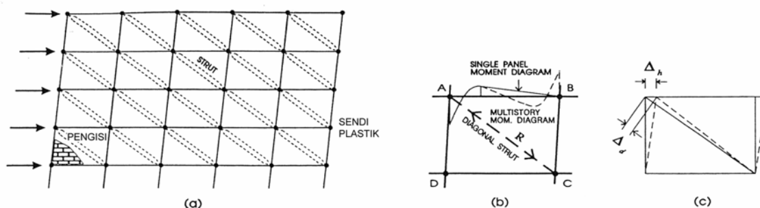
Gambar 5. Portal-berpenopang-ekvivalen
