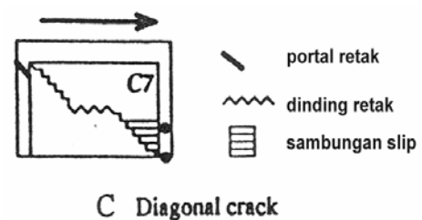
Gambar 3. Kondisi keruntuhan sampel uji portal-isi
