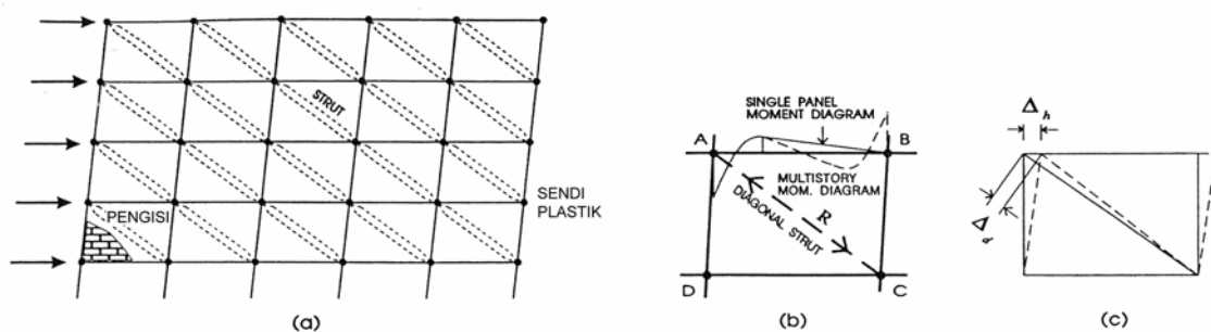
Gambar 5. Portal-berpenopang-ekvivalen
