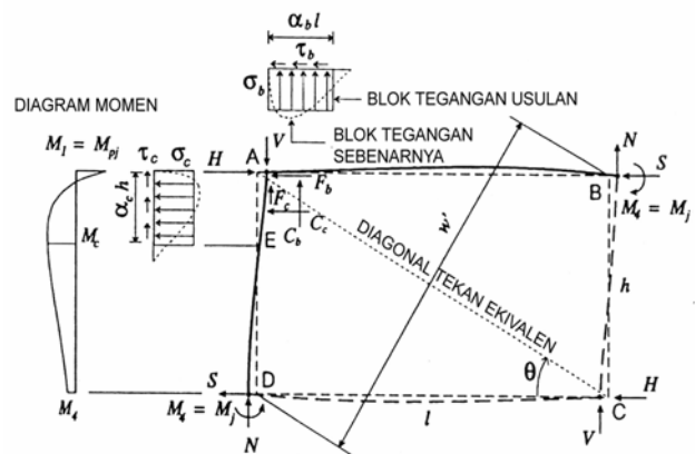
Gambar 6. Keseimbangan gaya pada portal-isi
