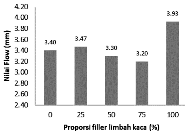
Gambar 2. Nilai flow pada kadar aspal optimum
