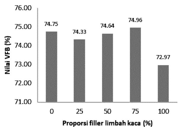
Gambar 6. Nilai VFB pada kadar aspal optimum
