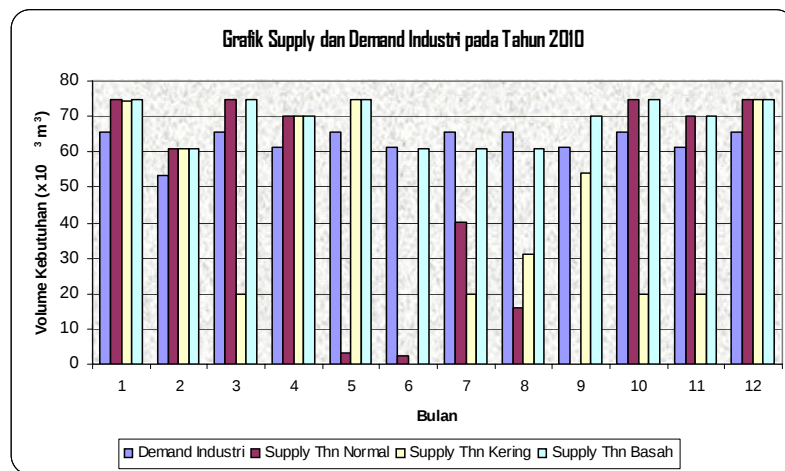
Gambar 17. Grafik supply dan demand industri pada tahun 2010
