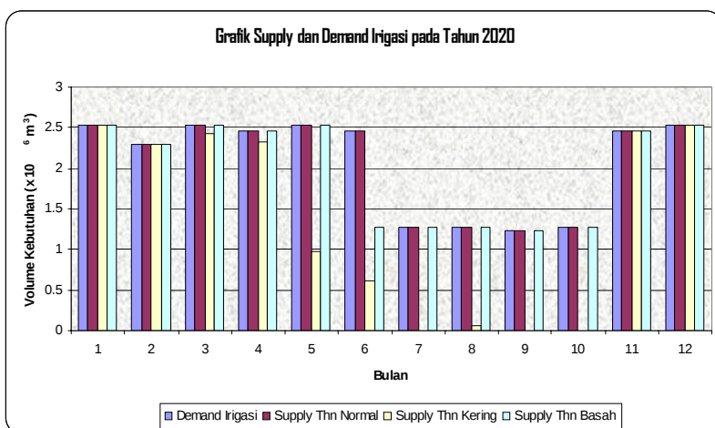
Gambar 18. Grafik supply dan demand irigasi pada tahun 2020
