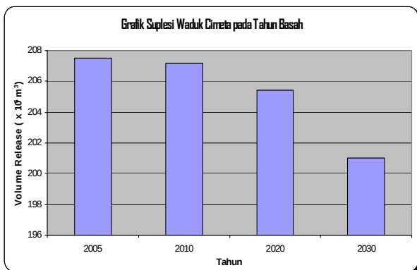
Gambar 26. Grafik suplesi Waduk Cimeta pada tahun basah
