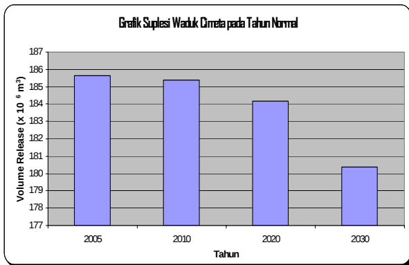
Gambar 25. Grafik suplesi Waduk Cimeta pada tahun normal
