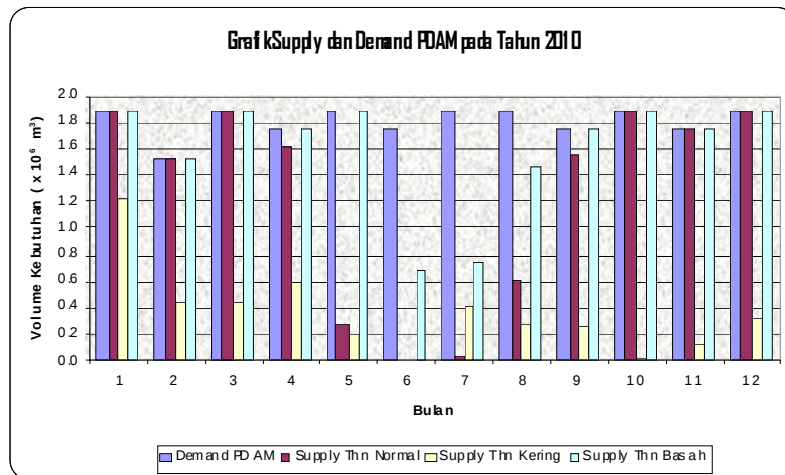
Gambar 16. Grafik supply dan demand PDAM pada tahun 2010
