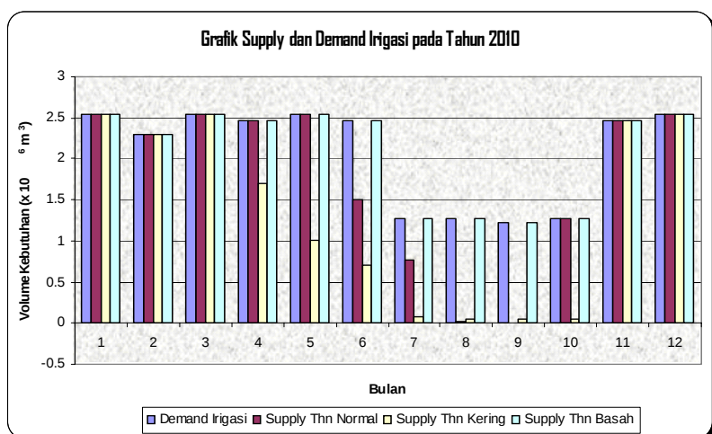
Gambar 15. Grafik supply dan demand irigasi pada tahun 2010
