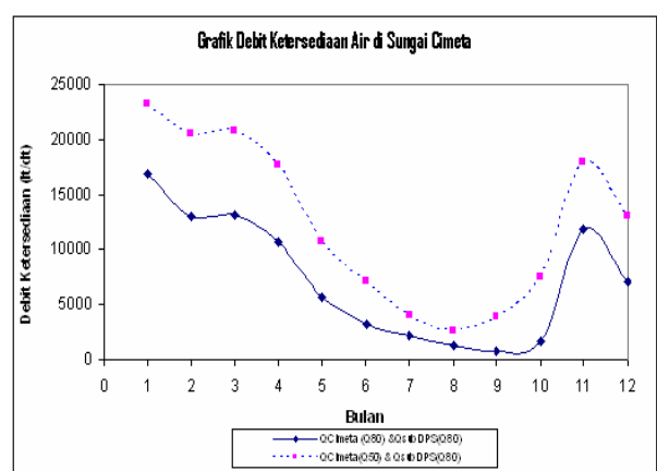
Gambar 3. Grafik debit ketersediaan air Sungai Cimeta
