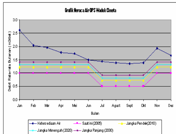
Gambar 6. Grafik neraca air DPS Waduk Cimeta
