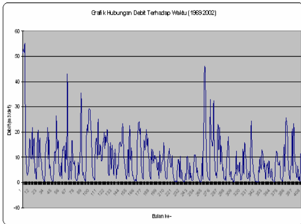
Gambar 4. Debit bulanan DPS Cimeta 34 tahun
