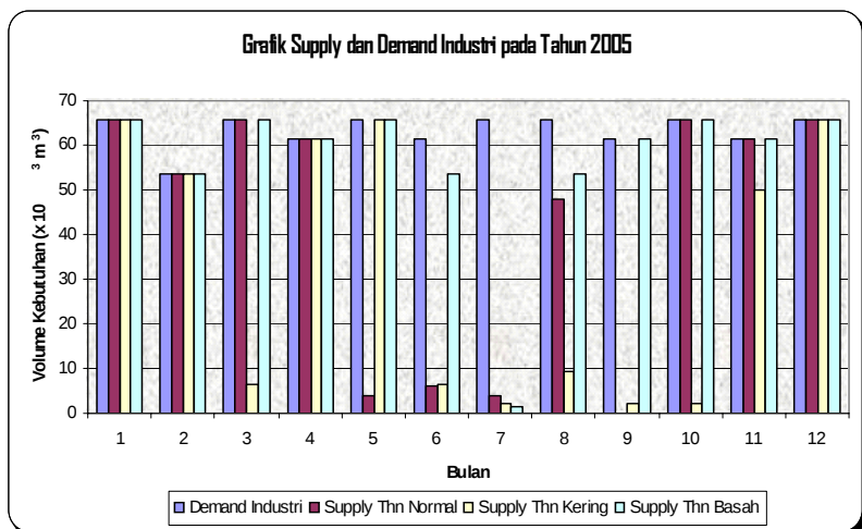
Gambar 14. Grafik supply dan demand industri pada tahun 2005
