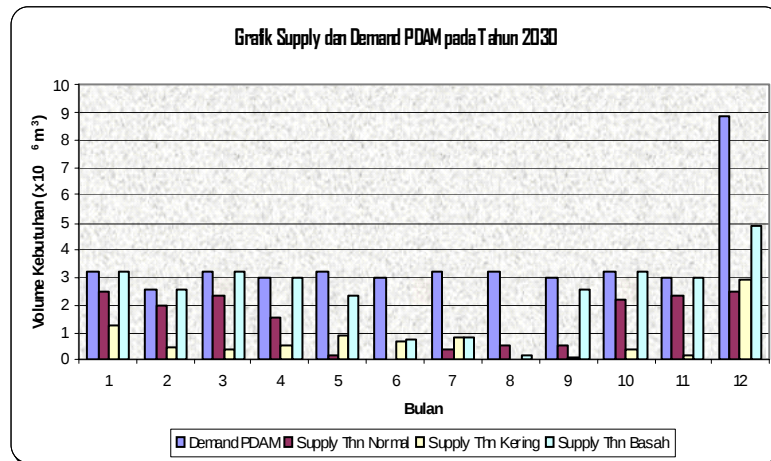
Gambar 22. Grafik supply dan demand PDAM pada tahun 2030
