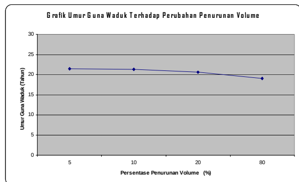
Gambar 28 Grafik umur guna waduk terhadap perubahan penurunan volume
