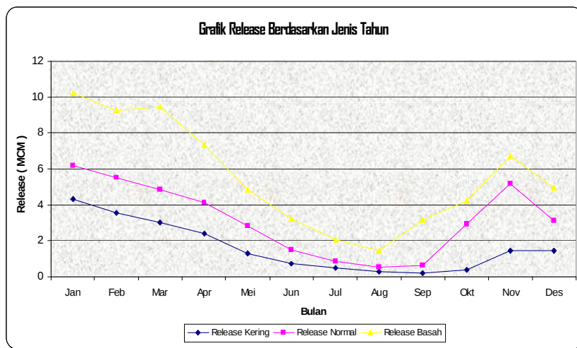
Gambar 11. Grafik release berdasarkan pada jenis tahun
