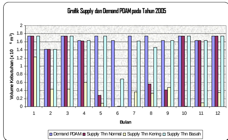
Gambar 13. Grafik supply dan demand PDAM pada tahun 2005
