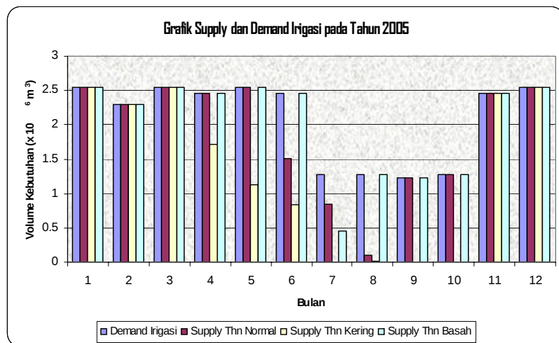
Gambar 12. Grafik supply dan demand irigasi pada tahun 2005
