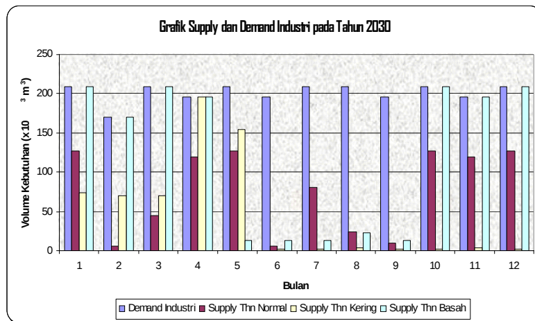
Gambar 23. Grafik supply dan demand Industri pada tahun 2030
