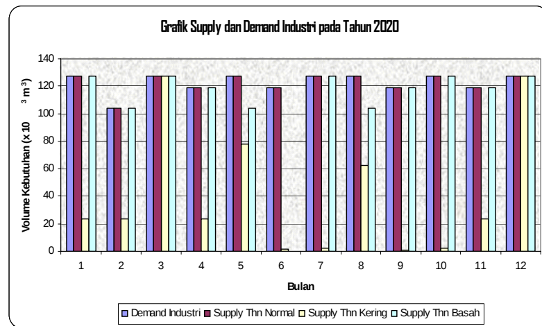
Gambar 20. Grafik supply dan demand industri pada tahun 2020
