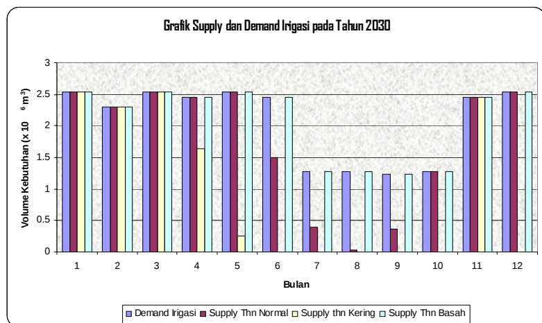
Gambar 21 Grafik supply dan demand irigasi pada tahun 2030
