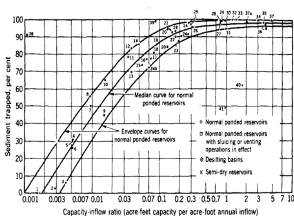
Gambar 2. Trap efficiency waduk sebagai fungsi dari rasio kapasitas inflow
