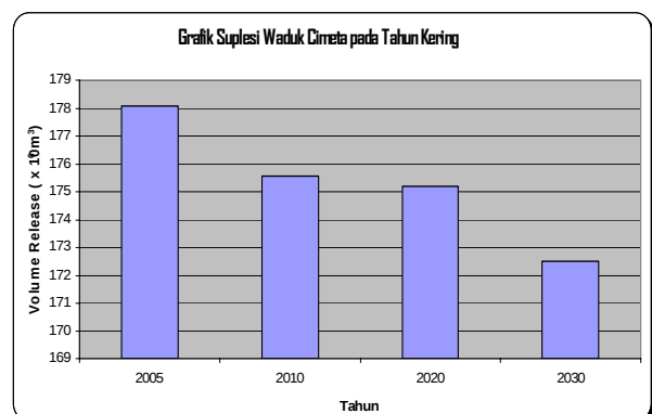
Gambar 24. Grafik suplesi Waduk Cimeta pada tahun kering
