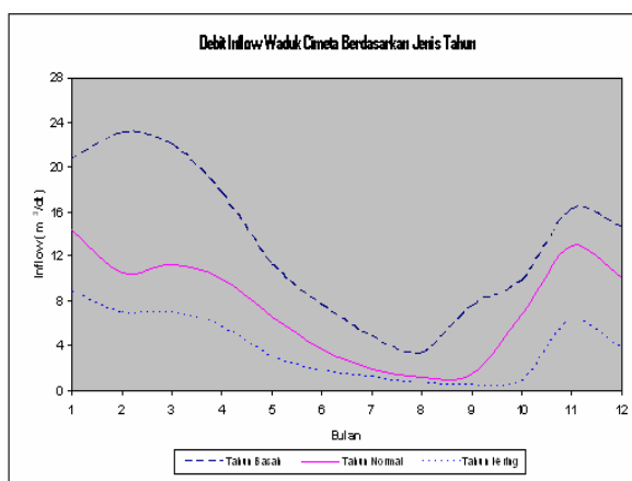
Gambar 7. Grafik debit inflow Waduk Cimeta berdasarkan jenis tahun
