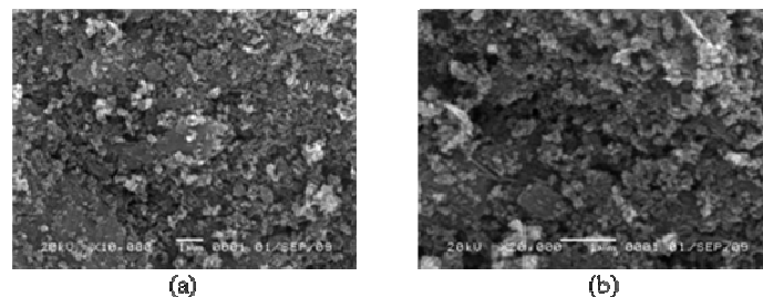
Gambar 5. Morfologi permukaan sampel fotokatalis \text{TiO}_2 -zeolit (20%). (a) pembesaran 10000 kali, (b) pembesaran 20000 kali
