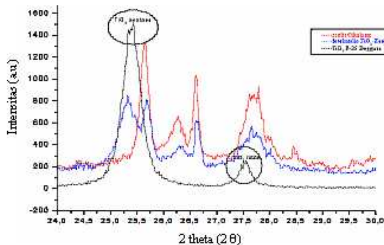
Gambar 3. Pola difraksi dari zeolit Cikalong, fotokatalis \text{TiO}_2 -zeolit (20%), dan standar \text{TiO}_2 P-25 Degussa setelah dipersempit skala pada 2\theta = 24^\circ - 30^\circ
